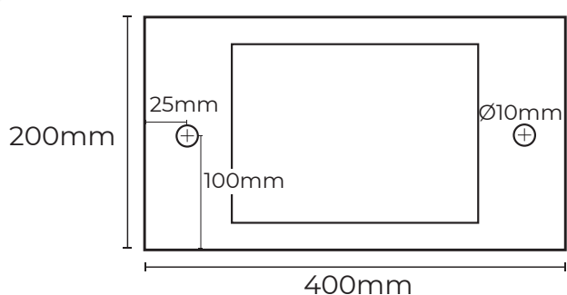
schema fori di fissaggio a terra
